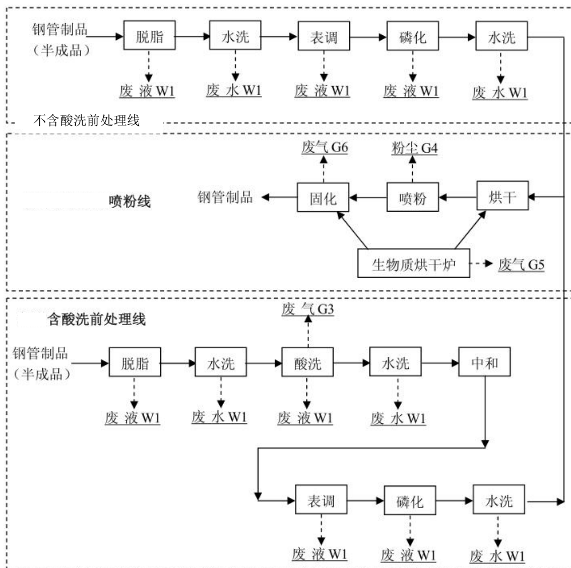
图 3.4-2 金属表面处理工艺流程及产污环节
