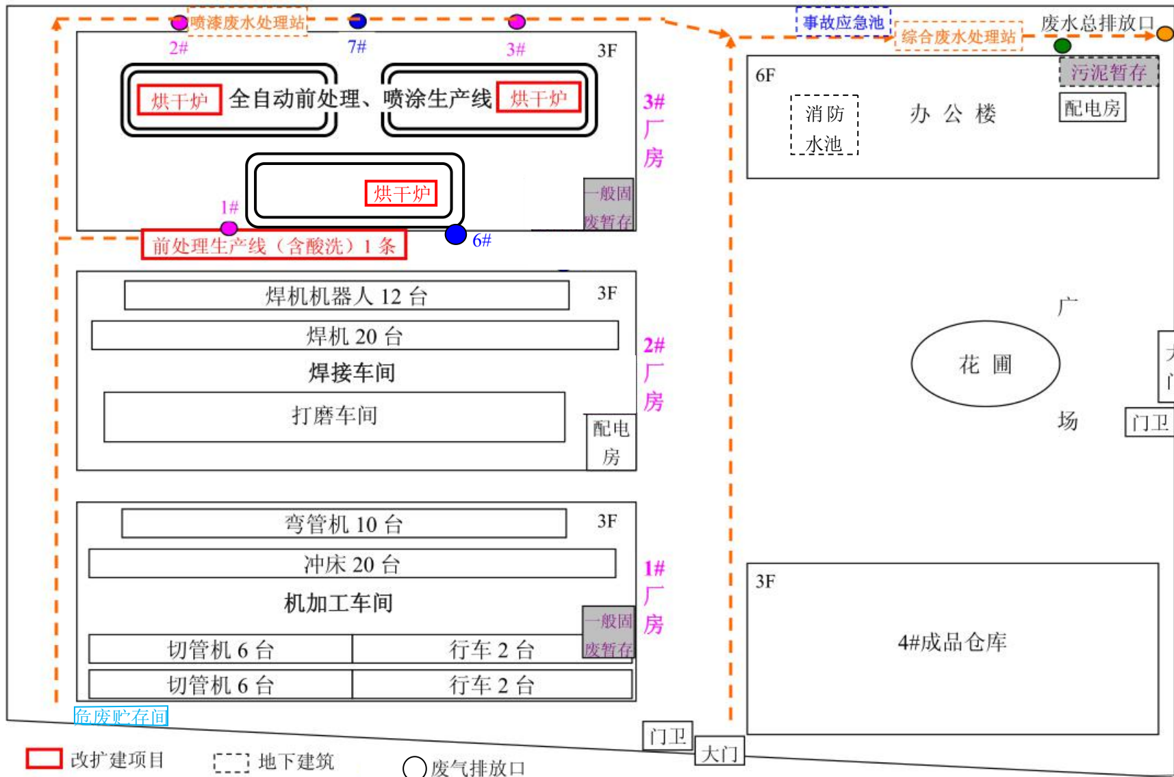
厂区平面布置图及厂房一层平面图
