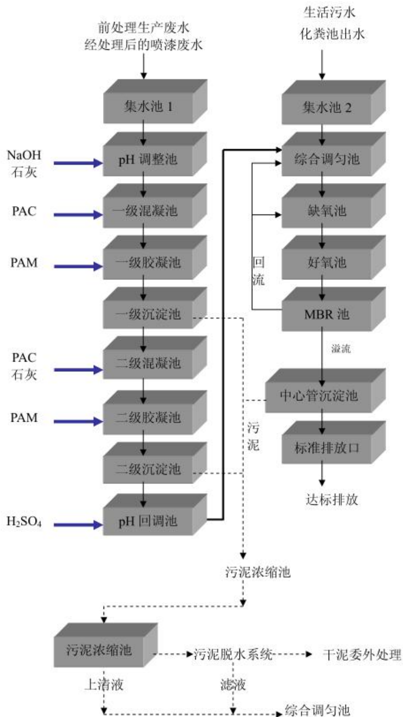
图 3.3-2 综合废水处理工艺流程图
