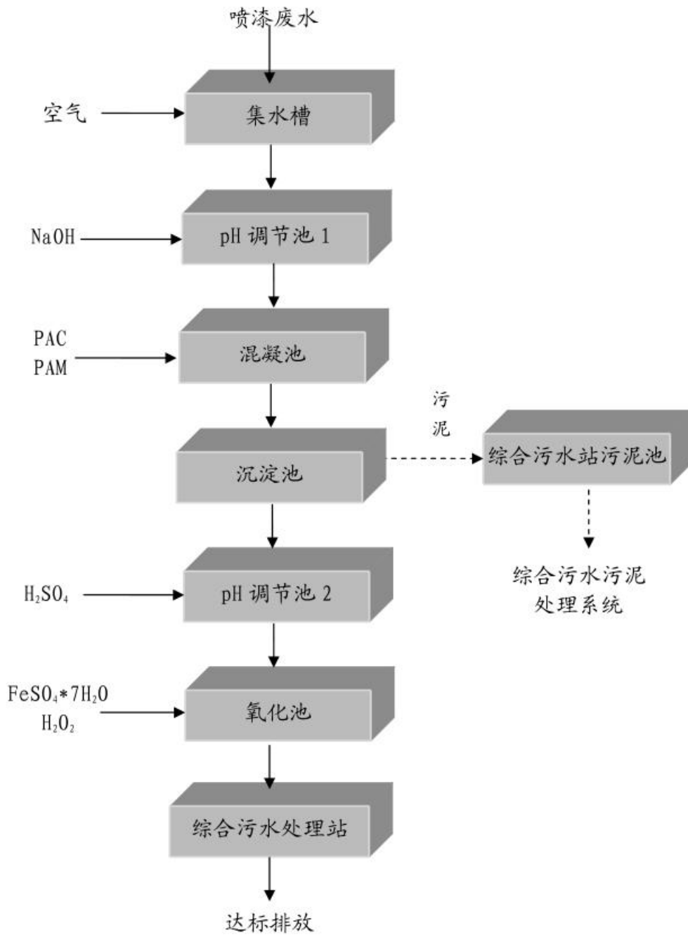
图 3.3-1 喷漆废水处理工艺流程图
