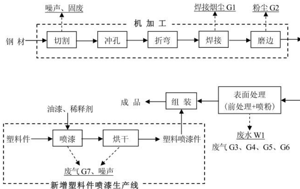
图 3.4-1 金属加工工艺流程及产污环节
